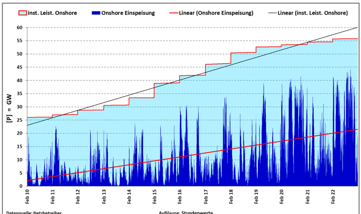
Abb. 55: Bilanz des Windkraftausbaus der letzten 12 Jahre
