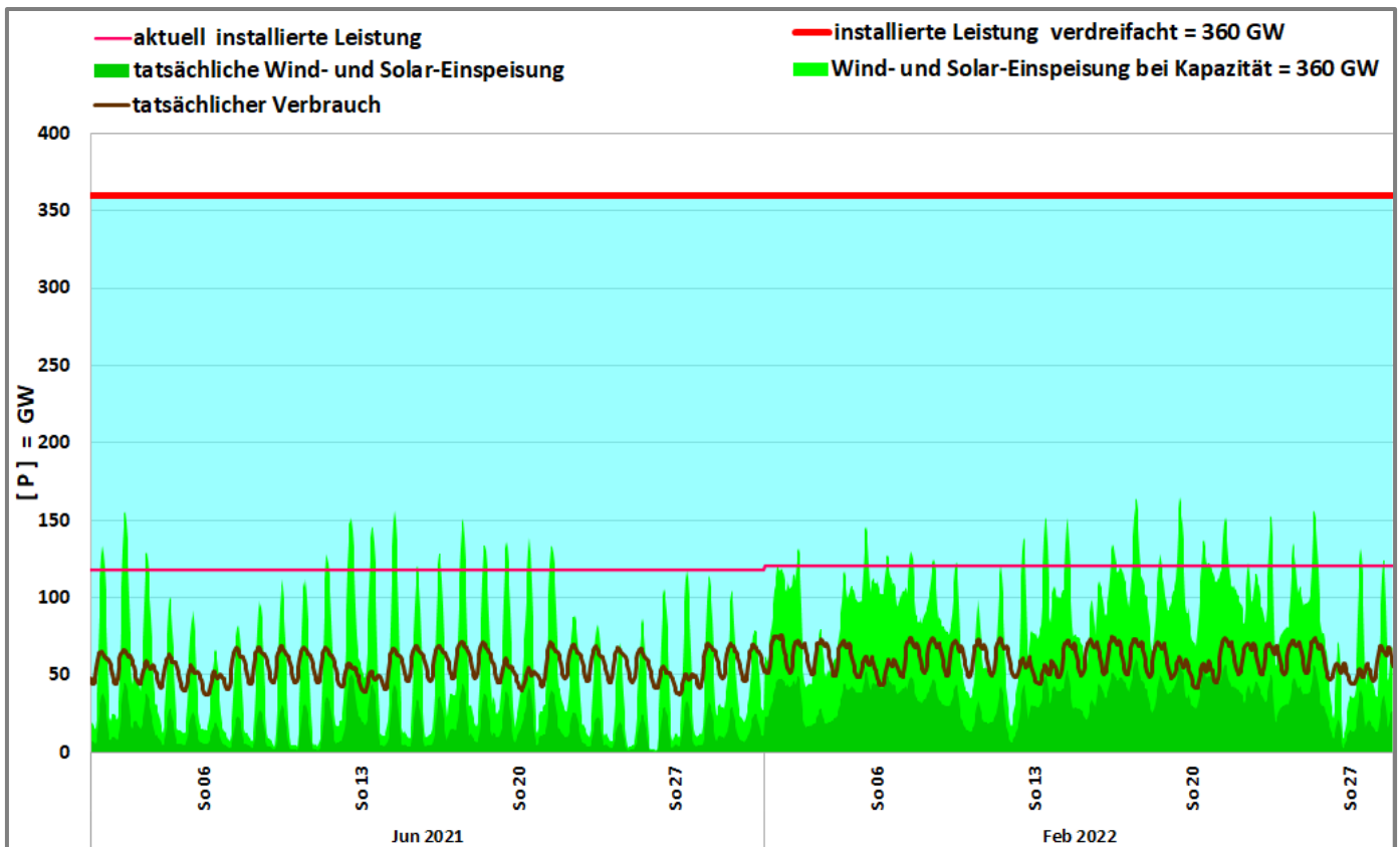
Abb. 54: Situation bei verdreifachten Wind- und Photovoltaikkapazitäten
